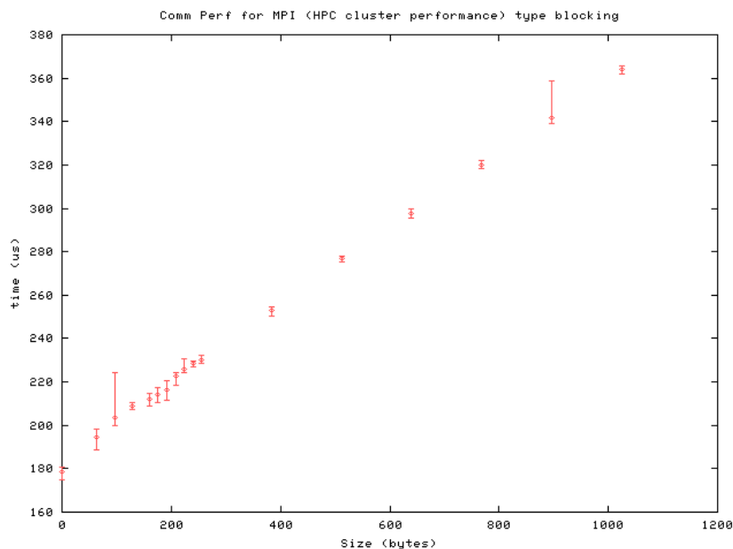
Figura 4.30: Prestazioni del cluster HPC con messaggi corti e protocollo sincro.
