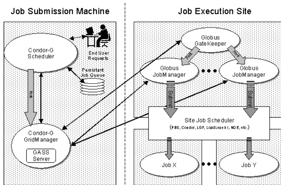
Figura 2.4: Esecuzione remota di Condor-G sopra risorse Globus.
